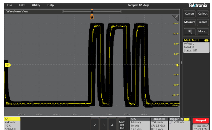
Grenzmaskentest basierend auf einem digitalen Referenzsignal
