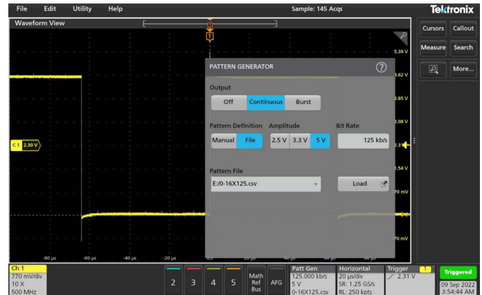
Digitale Bitmuster-Generator
