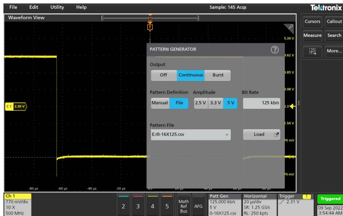
Digitaler Mustergenerator
